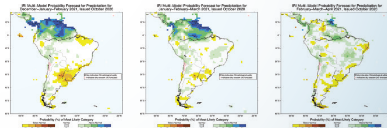
Figura 6 – Previsão climática para os trimestres dezembro-janeiro-fevereiro de 2020/21 a fevereiro-março-abril de 2021, de acordo com o IRI. Fonte: IRI ( https://iri.columbia.edu/our-expertise/climate/forecasts/seasonal-climate-forecasts/ ).
