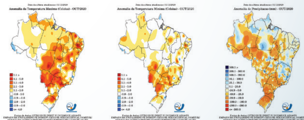
Figura 1 – Anomalias das temperaturas médias das máximas (Tmax, Esquerda) e das mínimas (Tmin, Centro) e da chuva acumulada (P, Direita) no mês de outubro de 2020 no Brasil. Fonte: CPTEC/INPE.
